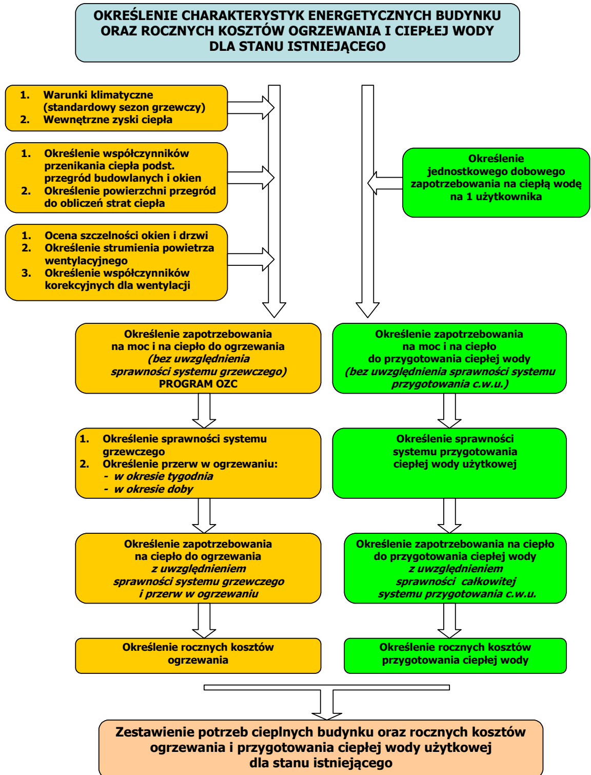
Rys. 3 Schemat określania charakterystyk energetycznych budynku oraz kosztów energii cieplnej dla stanu istniejącego
